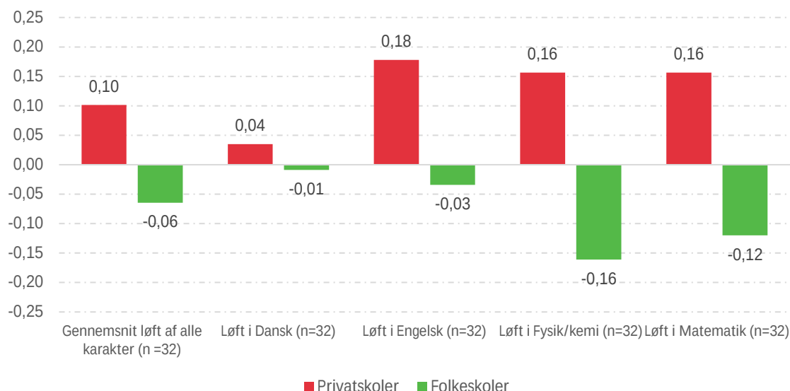
Figur 10 Gennemsnitlig undervisningseffekt for privatskoler og folkeskoler ved de afsluttende prøver i dansk, engelsk, fysik/kemi og matematik (skoler med op til ½ point forskel i social profil)
